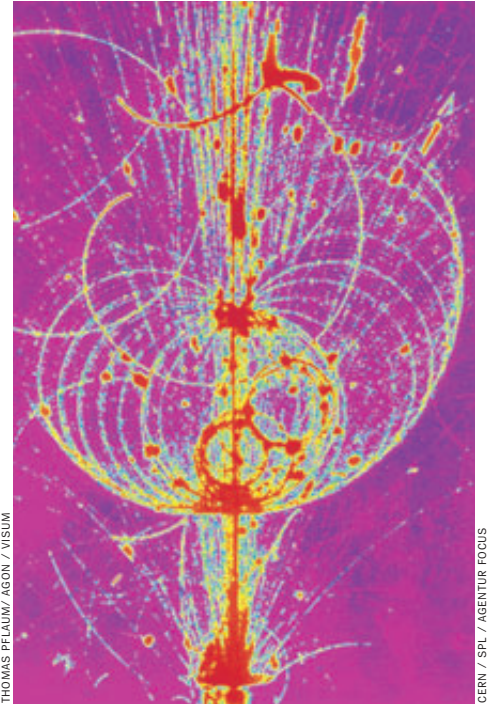
Teilchenbeschleuniger am Cern (in Genf), Kollisionsspuren: „Der wahre Grund lag darin, sich gegen neuartige Waffen zu versichern“
